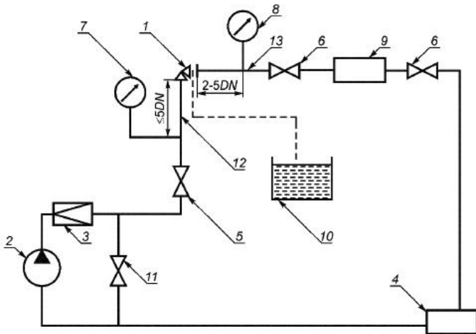
а) схема стенда для испытания арматуры с корпусами проходными (с патрубками на одной оси и со смещенными осями патрубков)
