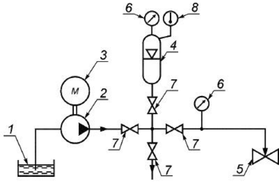
Рисунок Б.4 - Рекомендуемая схема стенда для количественного определения утечек в затворе арматуры с применением манометрического метода контроля (способ реализации метода - компрессионный)
